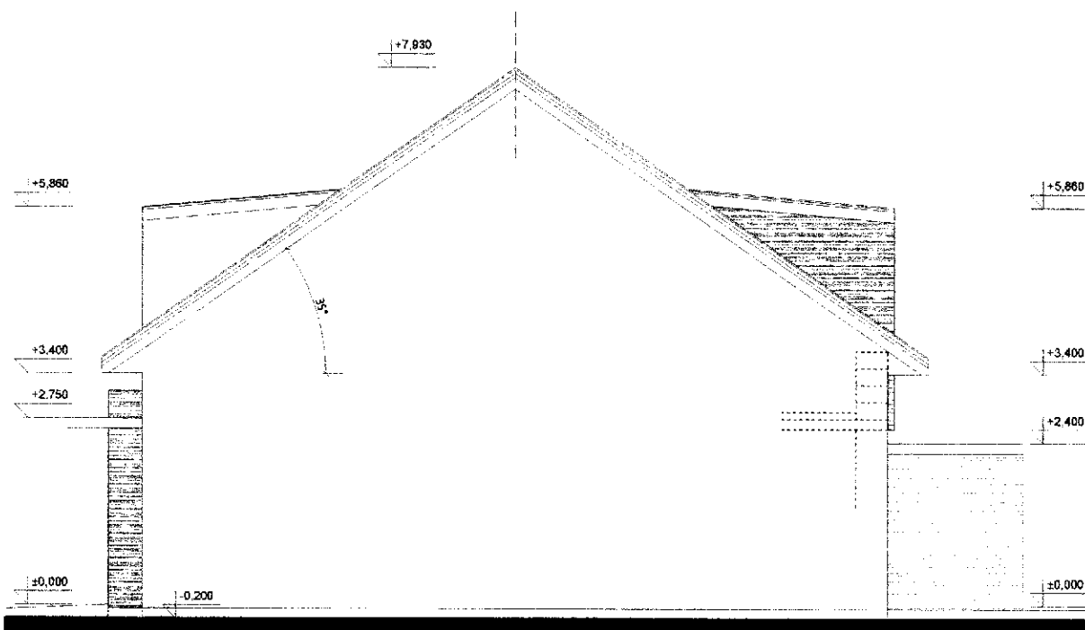
POHLED ZÁPADNÍ M1:100
