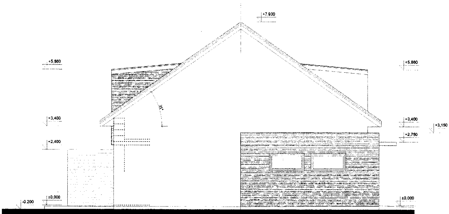
POHLED VÝCHODNÍ M1:100
