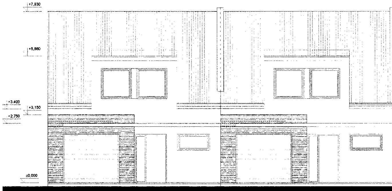
POHLED SEVERNÍ (OD ULICE ) M1:100
